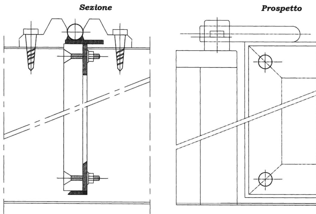
Tavola 1 - Particolare della testata oscillante
